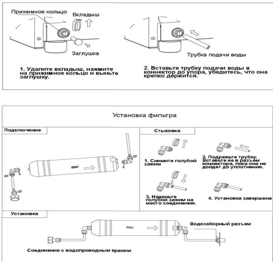
Рис.2 Схема подключению к водоснабжению.
